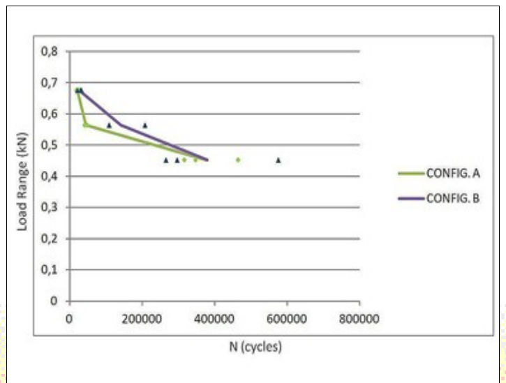
Figuur 8: Wöhlercurves van twee verschillende configuraties met drie clinchverbindingen
